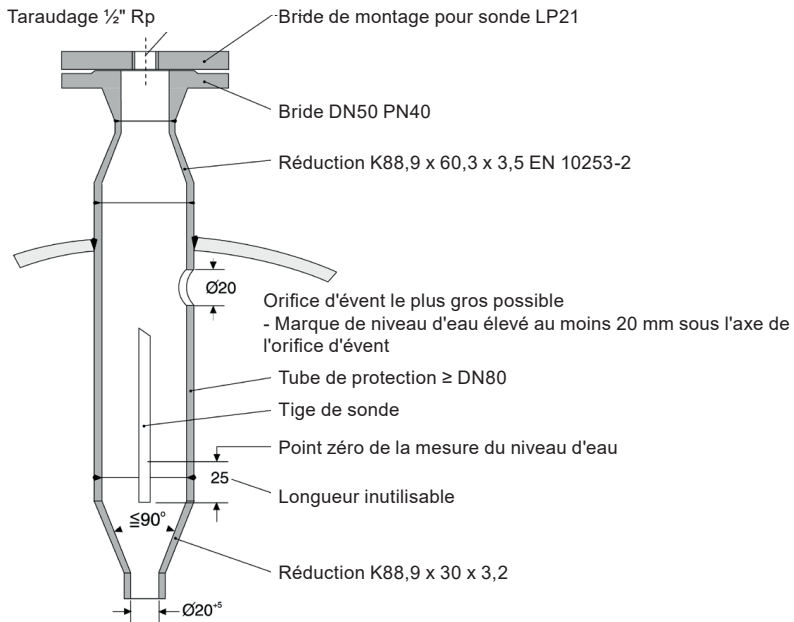
Fig.3 - Exemple d'installation 1 : à l'intérieur de la chaudière avec bouteille de protection fourni par le client
