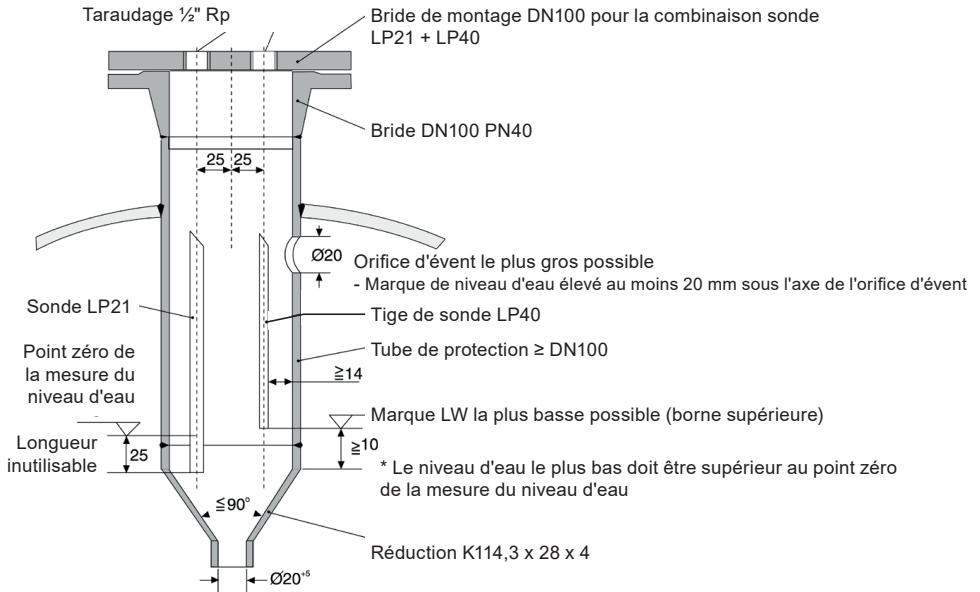
Fig.4 - Exemple d'installation 2 : Combinaison avec sonde limiteur de niveau d'eau LP40
