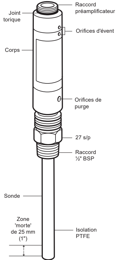
Fig. 1 - Sonde capacitive de niveau
