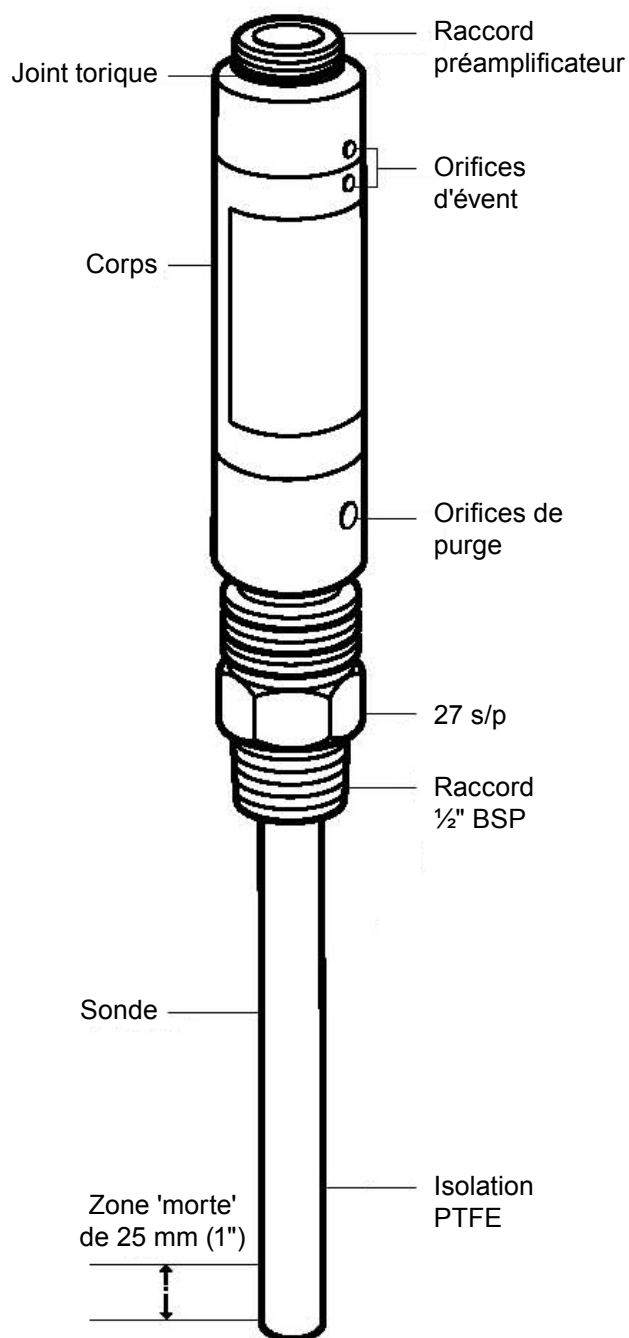
Fig. 1 Sonde de niveau
