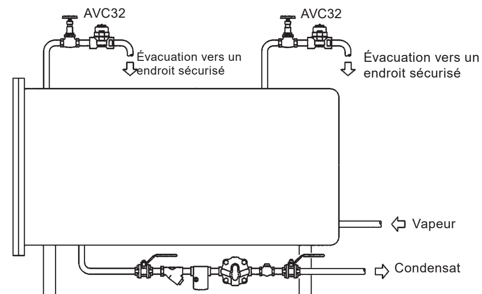
Fig. 2 - Bout de ligne d'une distribution principale
