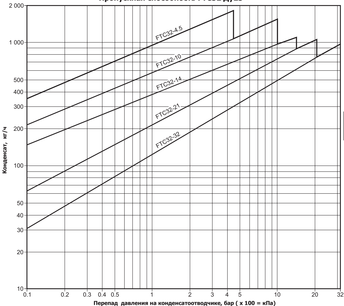
Пропускная способность FTC32 Ду25
