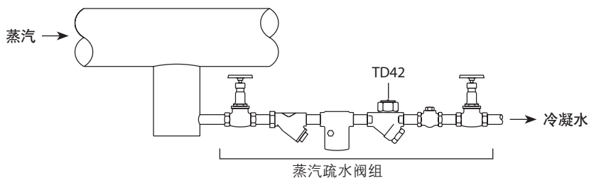
图2 典型应用
