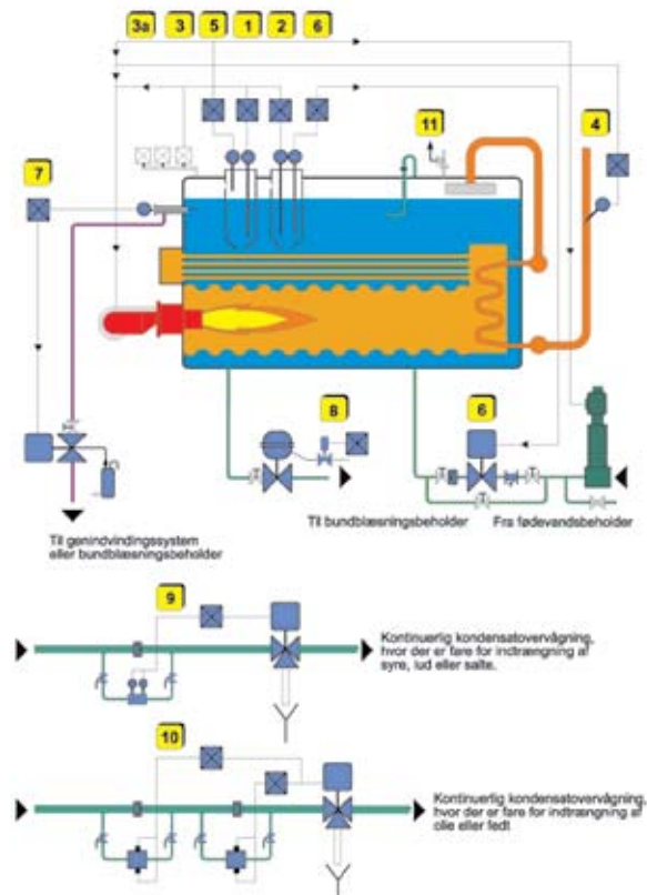
Dampkedler efter TRD 604 - 72 timers periodisk overvågning Udstyr til dampkedler.
