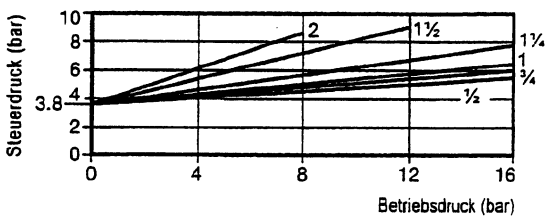
PF_1G-3BD - Anströmung über Ventilsitz (1 nach 2)
