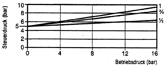
PF_1G-2BD - Anströmung über Ventilsitz (1 nach 2)
