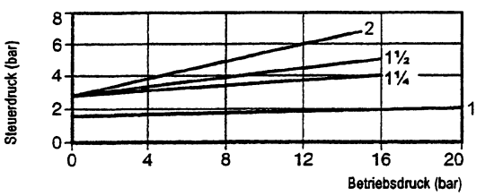
PF61G-3 NC - Anströmung über Sitz
