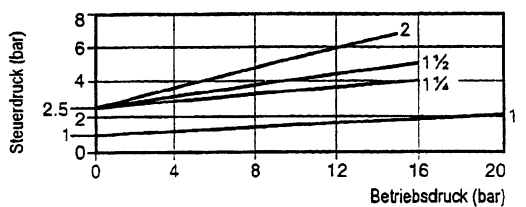
PF51G-3NC - Anströmung über Sitz
