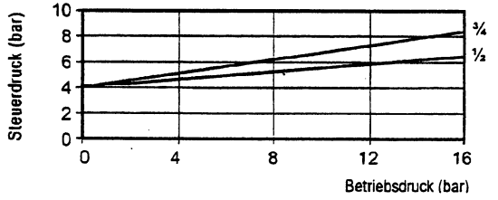
PF51G-1BD - Anströmung über Ventilsitz (1 nach 2)
