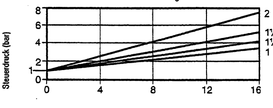
PF 61G-3 NO / PF 51G-3 NO - Anströmung unter Sitz
