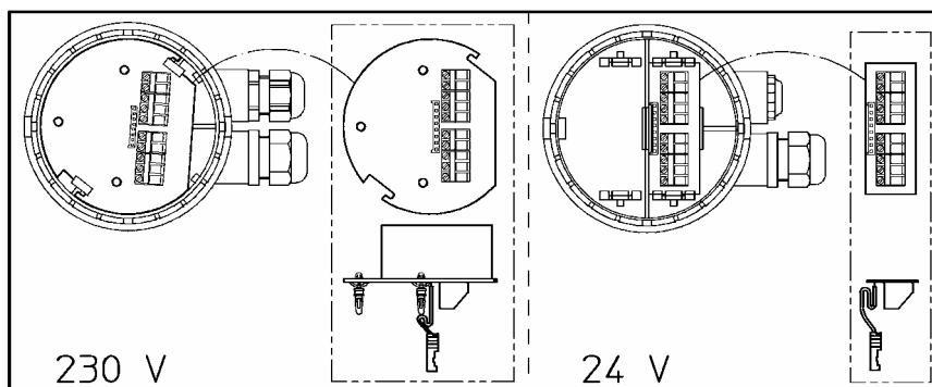
Bild 5: Herausnahme der Klemmleiste
