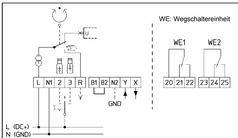
Bild 7: Schaltplan für MC 163_230 und MC 163_24
