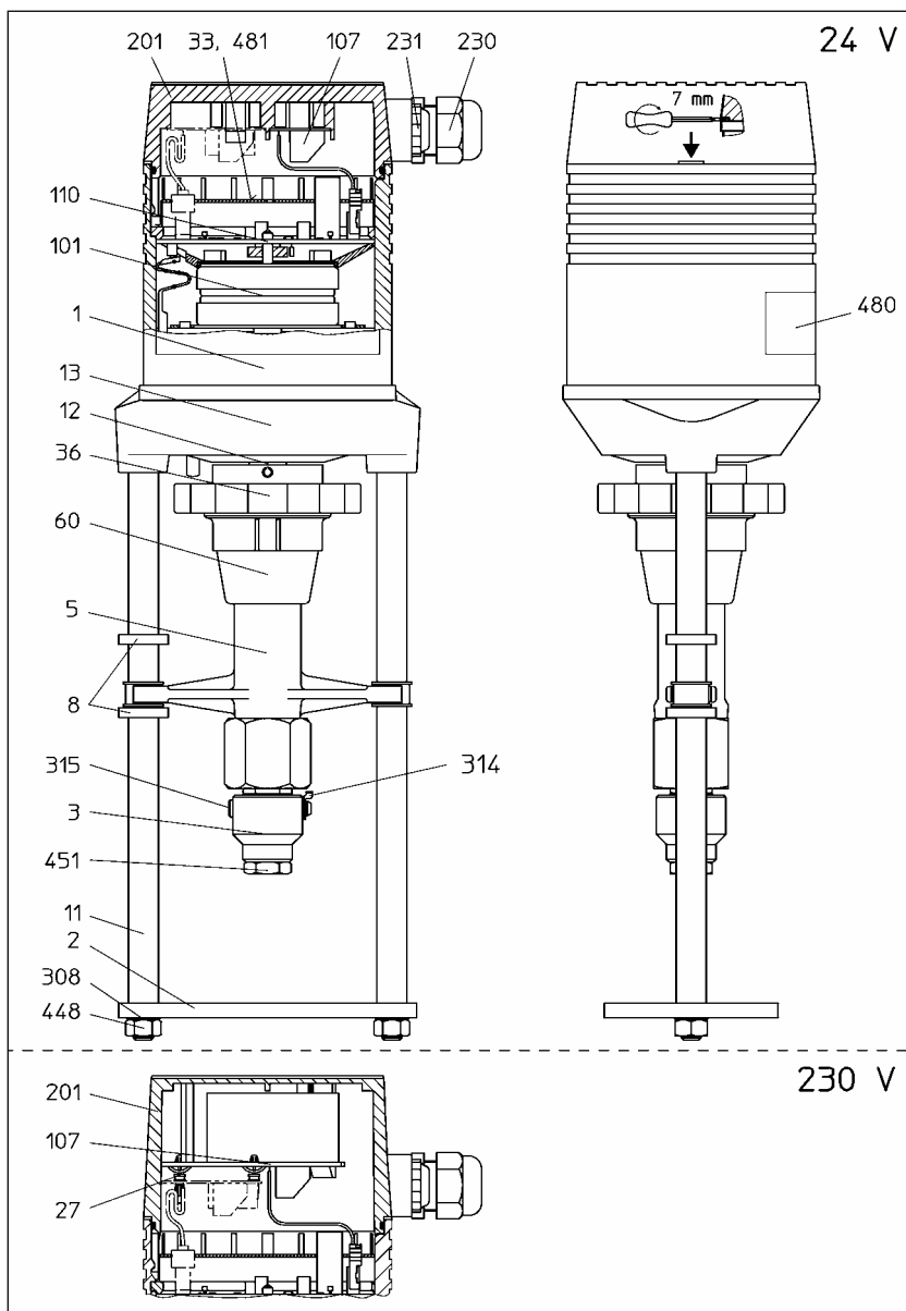
Bild 14: Schnittzeichnung mit Positionierung von Einzelteilen für Typ MC163_24 und MC163_230.
