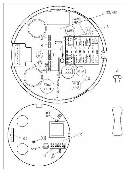
Bild 8: Abdeckung (33) der Hauptplatine (110).
