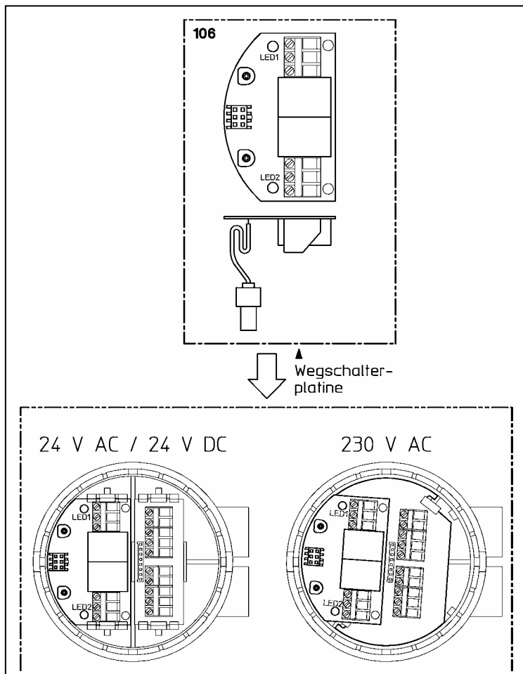
Bild 10: Einbau der Wegenschalter
