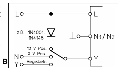
Bild 6: Diodenschaltung
